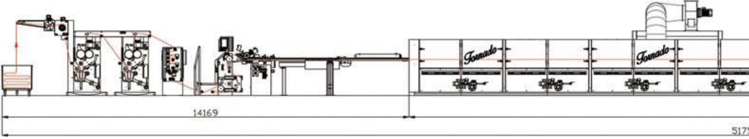
Örgü Hattı; Tek Taraftan Hava Sirkülasyonu, Dik veya Yatık tip zincir sistemi
