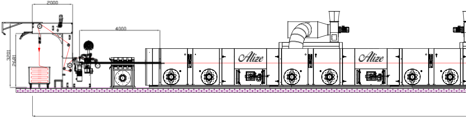
Örgü Hattı; Çapraz Hava Sirkülasyonu, Dik veya Yatık tip zincir sistemi
